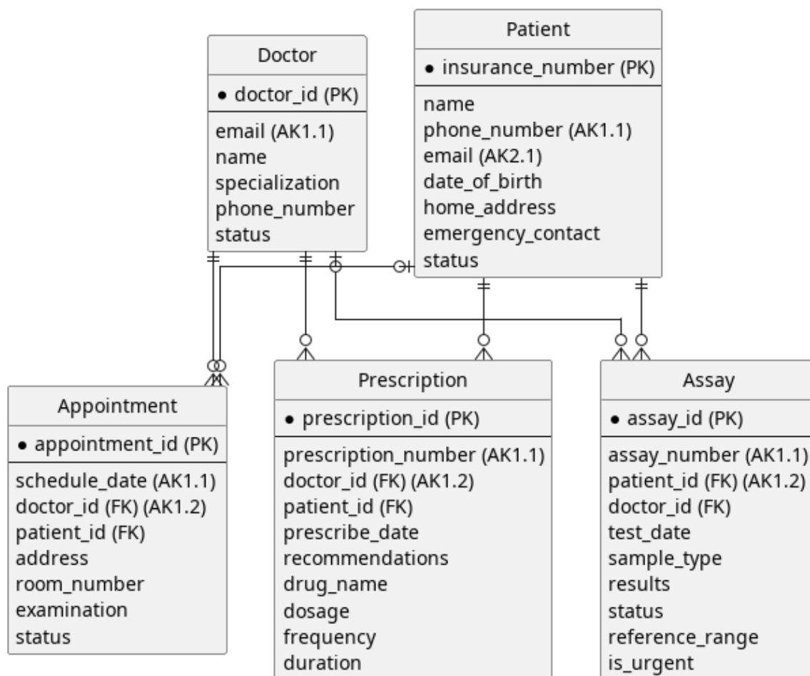
Рис. 3 — Реляционная модель системы «Поликлиника», полученная из модели «сущность-связь»
