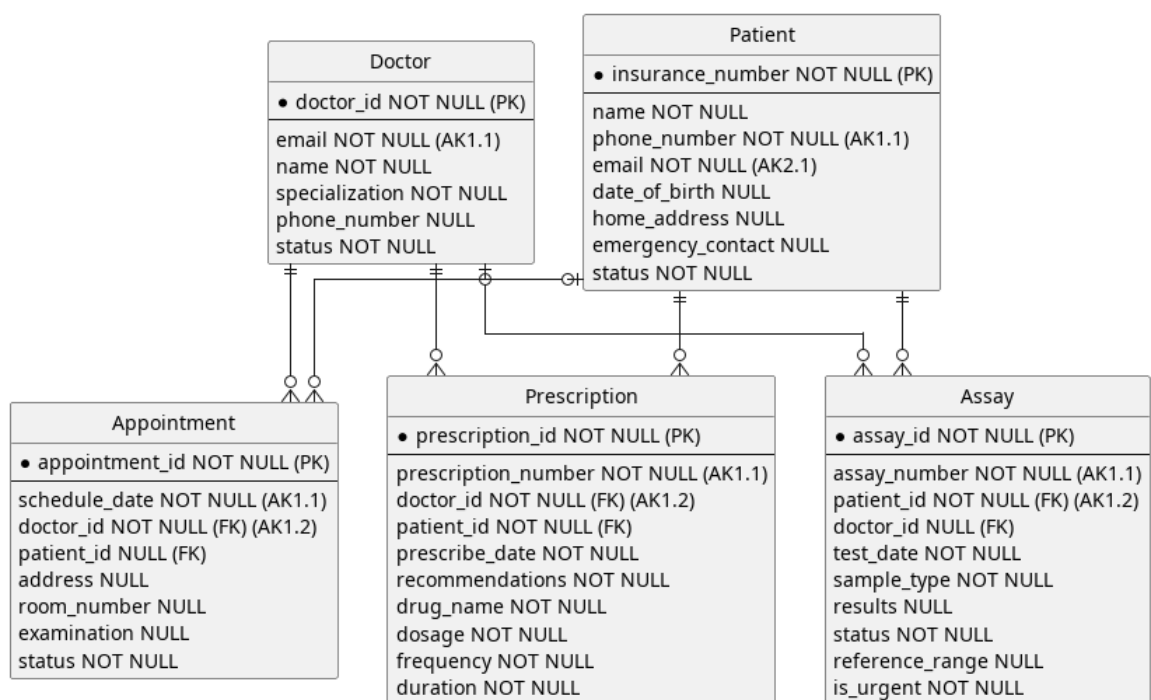
Рис. 2 — Реляционная модель системы «Поликлиника», полученная из семантической модели
