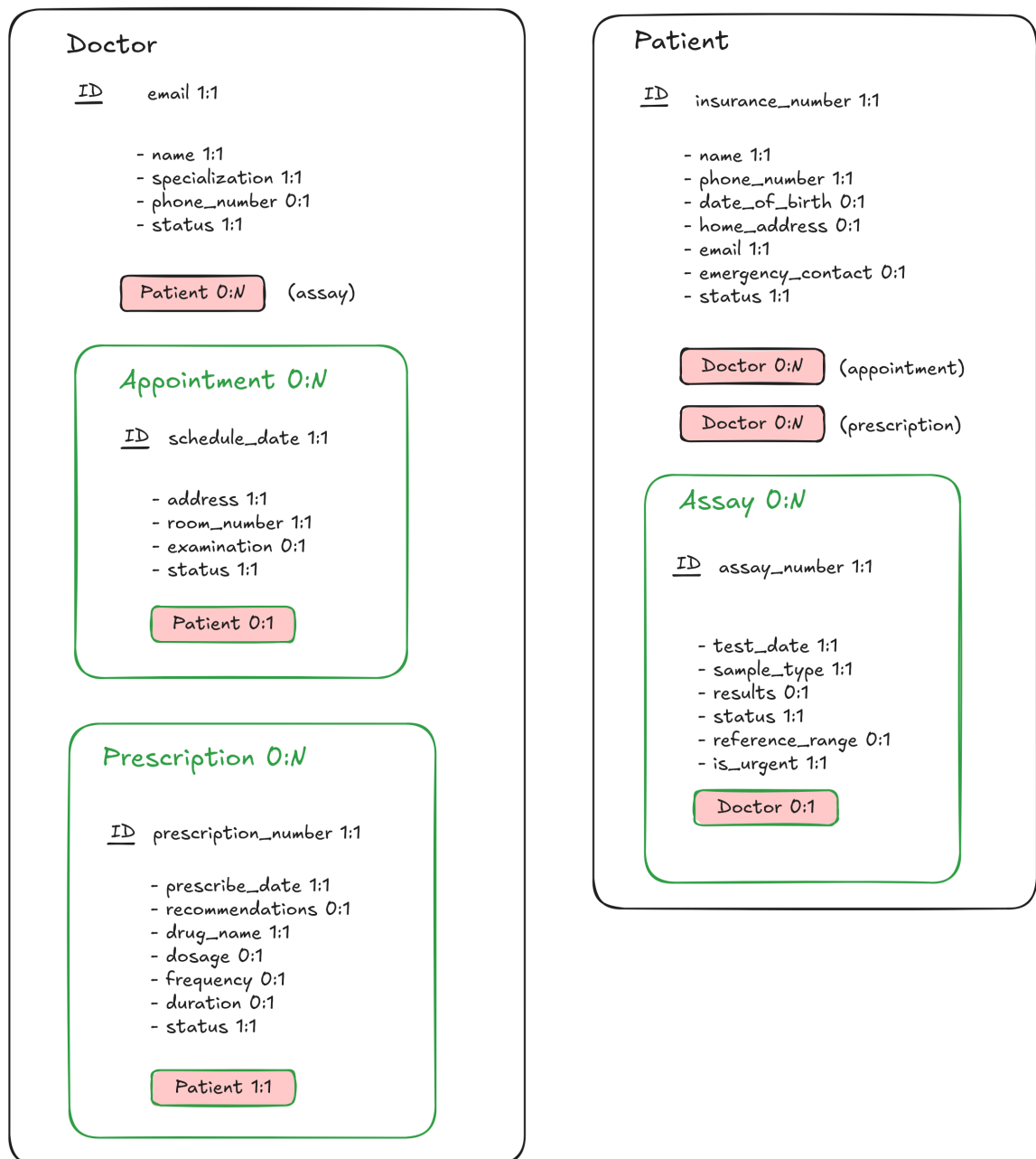
Рис. 1 — Семантическая модель системы «Поликлиника»
